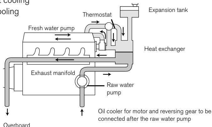
Keel cooling
